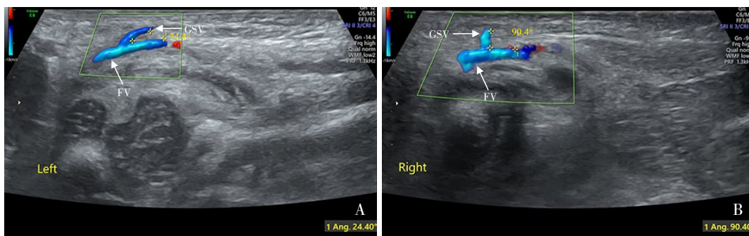
图 1 超声监测指导下肢静脉血管选择 图 A 显示 GSV 与 FV 夹角较小 (24.4°), 图 B 显示 GSV 与 FV 夹角较大 (90.4°)。GSV 与 FV 夹角越小导管越容易通过, 因此选择图 A 所示 GSV 置管。[GSV] 大隐静脉; [FV] 股静脉。
